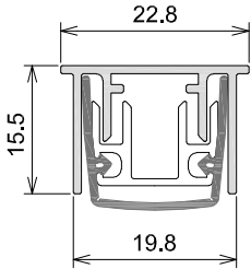
BOD50...
