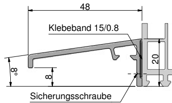
WS4820/SK
