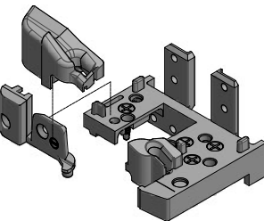
SH882-8020
