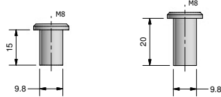
HÜ81515/si.
