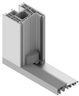
SCHWELLENHALTER
